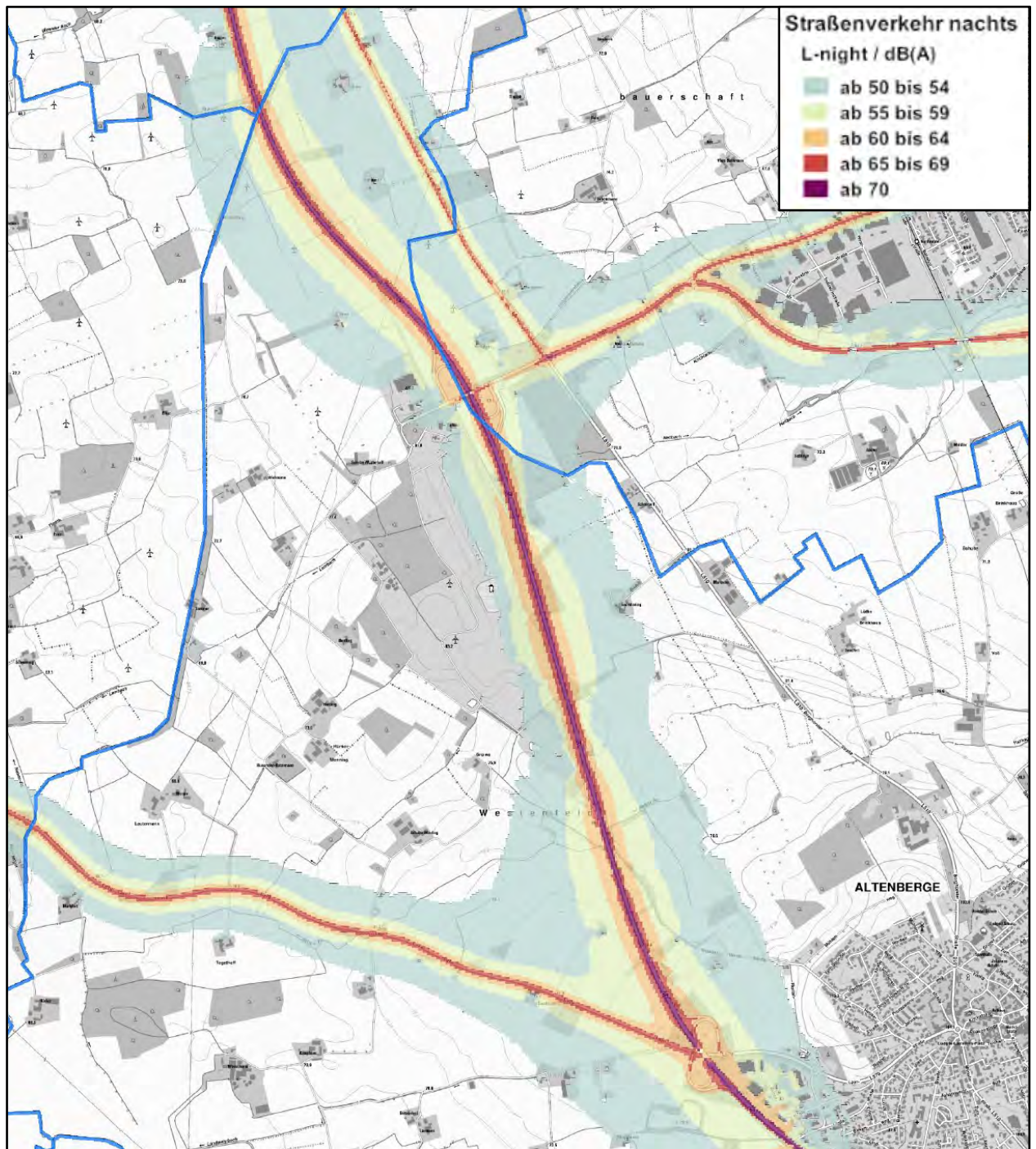
Karte 2: Isophonenkarte Nacht L_{night} für nördlich von Altenberge, genordet, ohne Maßstab (Auszug aus Anlage 3)
