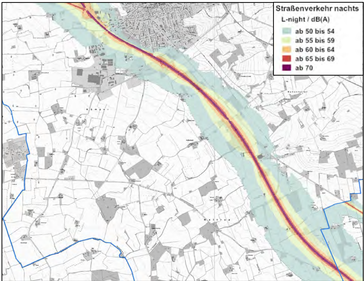
Karte 4: Isophonenkarte Nacht L_{\text{night}} für südlich von Altenberge, genordet, ohne Maßstab (Auszug aus Anlage 5)
