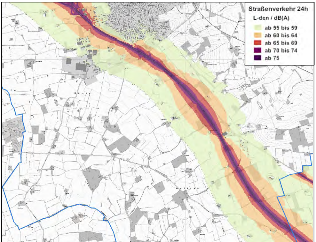
Karte 3: Isophonenkarte Tag L_{den} für südlich von Altenberge, genordet, ohne Maßstab (Auszug aus Anlage 4)
